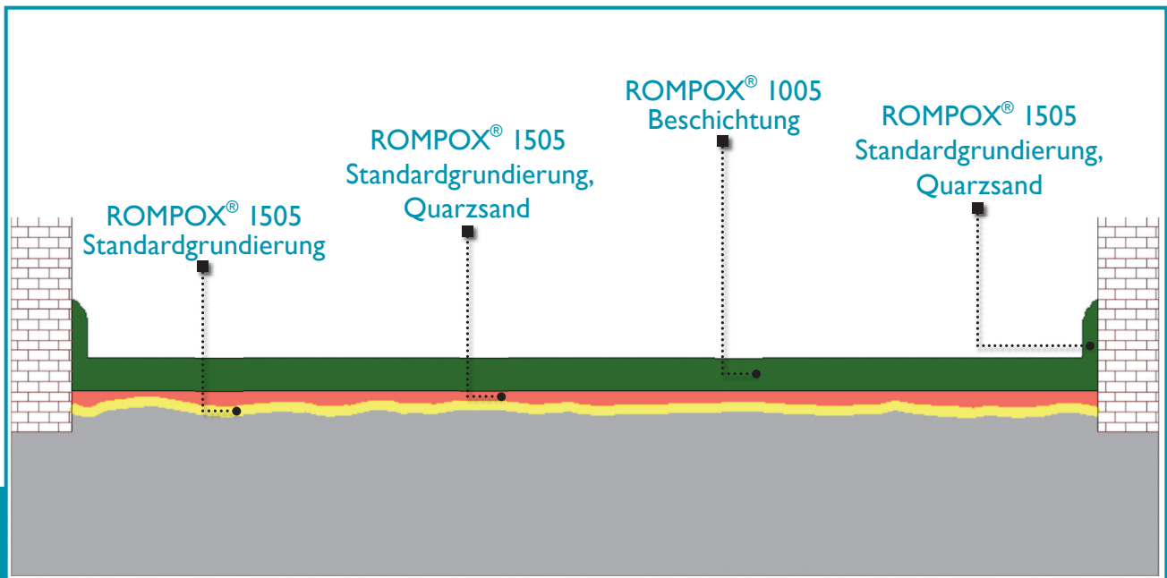
Systemaufbau - "Bodenbeschichtung"
