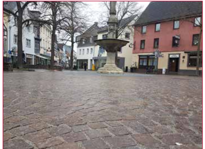
Für die Gesamtverfugung wurde mit 2 Arbeitern 5 Tage benötigt The entire jointing was done in 5 days with 2 workers
